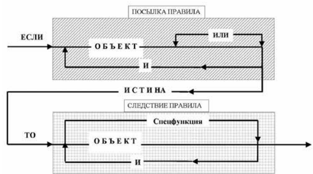
Рис. 3. Синтаксическая диаграмма
